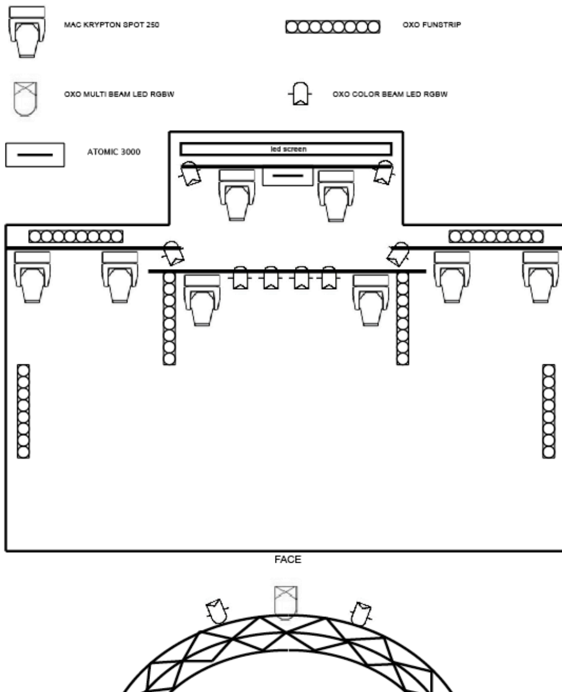
PLAN DE FEU BUS PALLADIUM - VUE DE DESSUS
